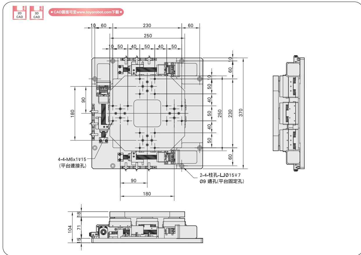
EXYY-025-025-42M 尺寸圖 Size
