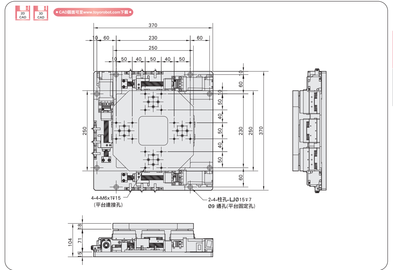
EXYY-025-025-M10 尺寸圖 Size
